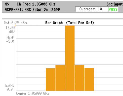
W-CDMA ACPR
