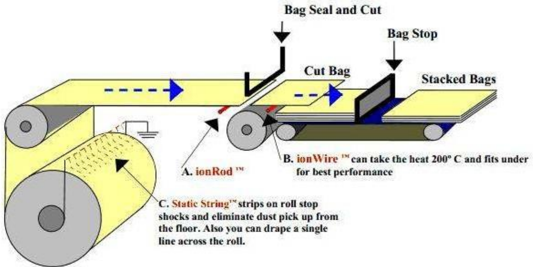
Sơ đồ vận hành Màng bao bì và những vị trí có thể phát sinh tĩnh điện
