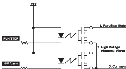
出力回路図 (フォトモスリレー出力)
