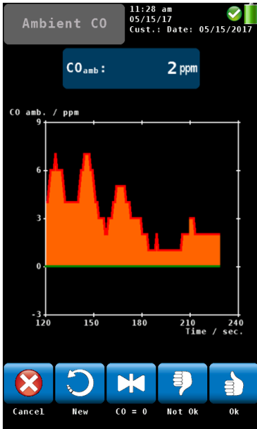
Fig. 21: Ambient CO
